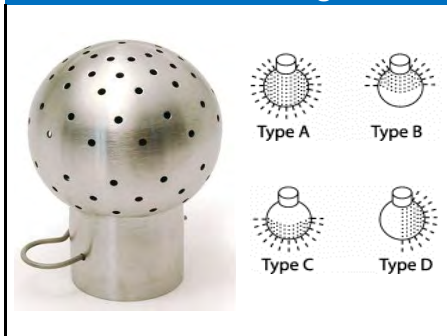
Boules de lavage
