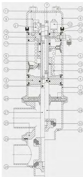
Joint métallique
